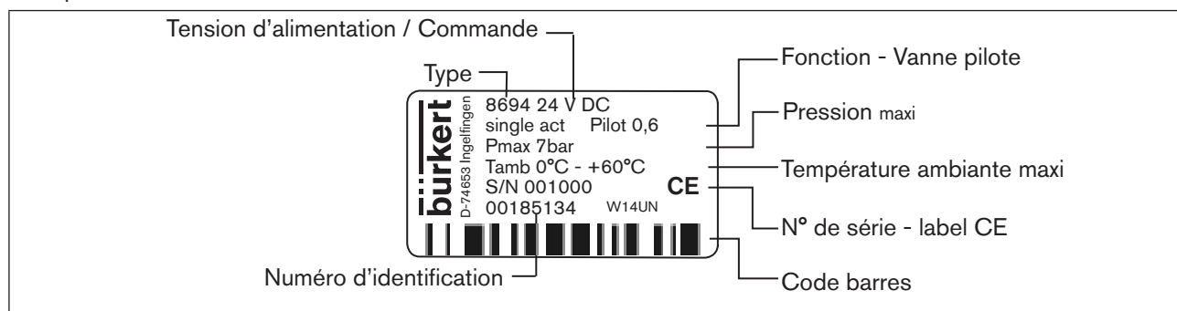
Figure 7 : Plaque signalétique (exemple)
