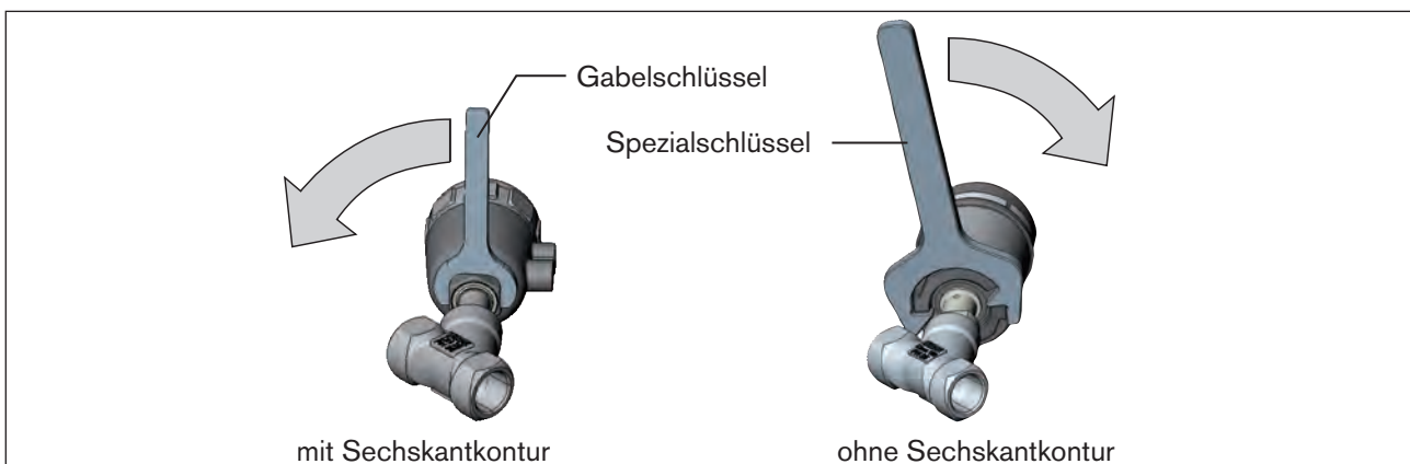
Bild 30: Drehen mit Speziesschlüssel / Gabelschlüssel
