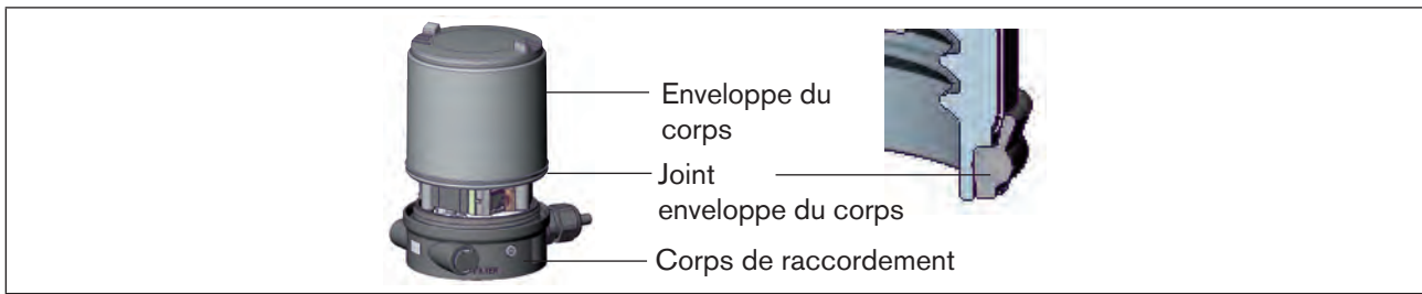
Figure 48 : Position du joint (enveloppe du corps)
