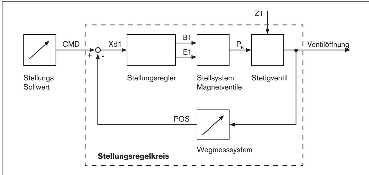
Bild 4: Signalfussplan Stellungsregler
