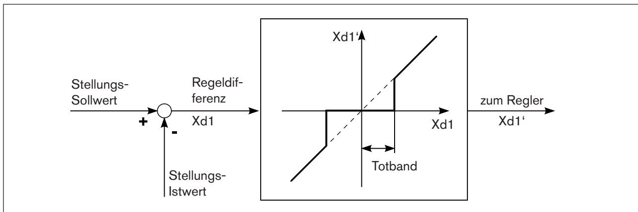
Bild 57: Diagramm X.CONTROL
