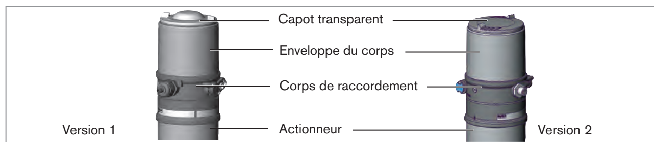
Figure 16 : Ouvrir positionneur
