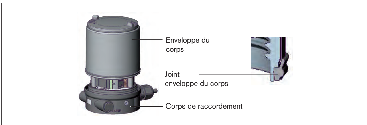
Figure 12 : Position du joint (enveloppe du corps)
