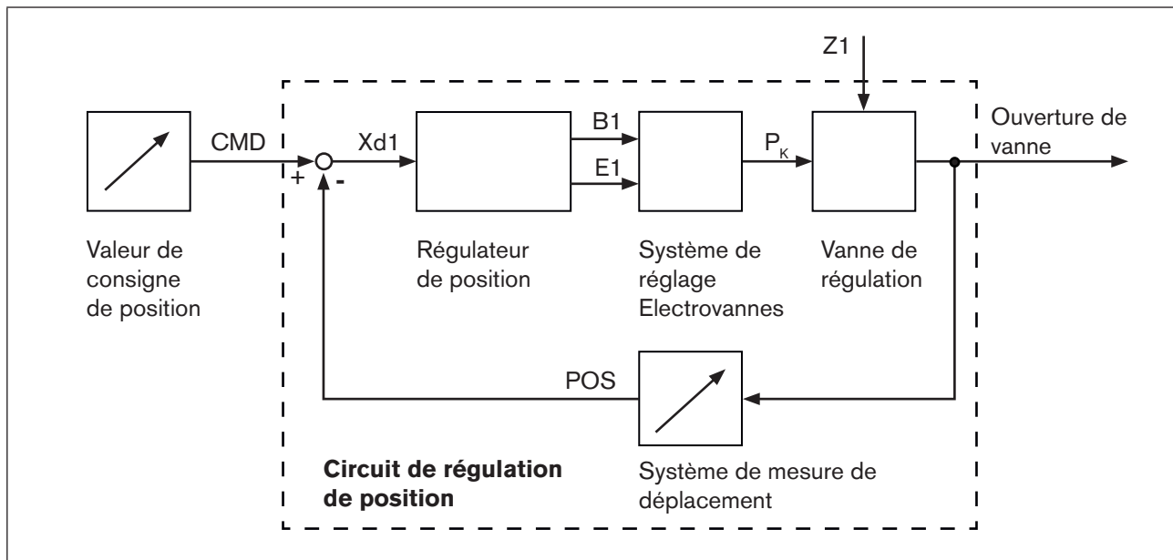
Figure 4 : Schéma logique du régulateur de position
