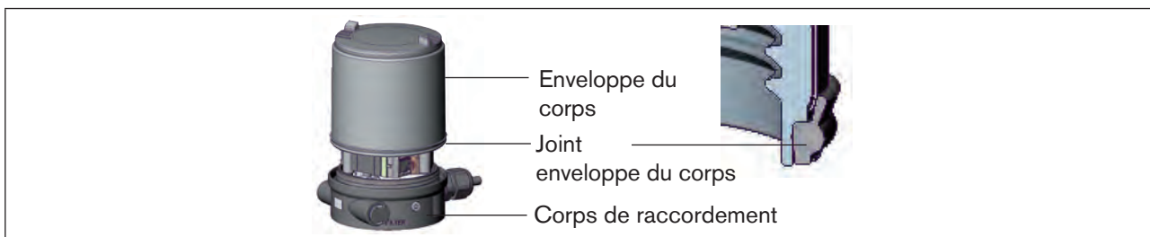
Figure 41 : Position du joint (enveloppe du corps)
