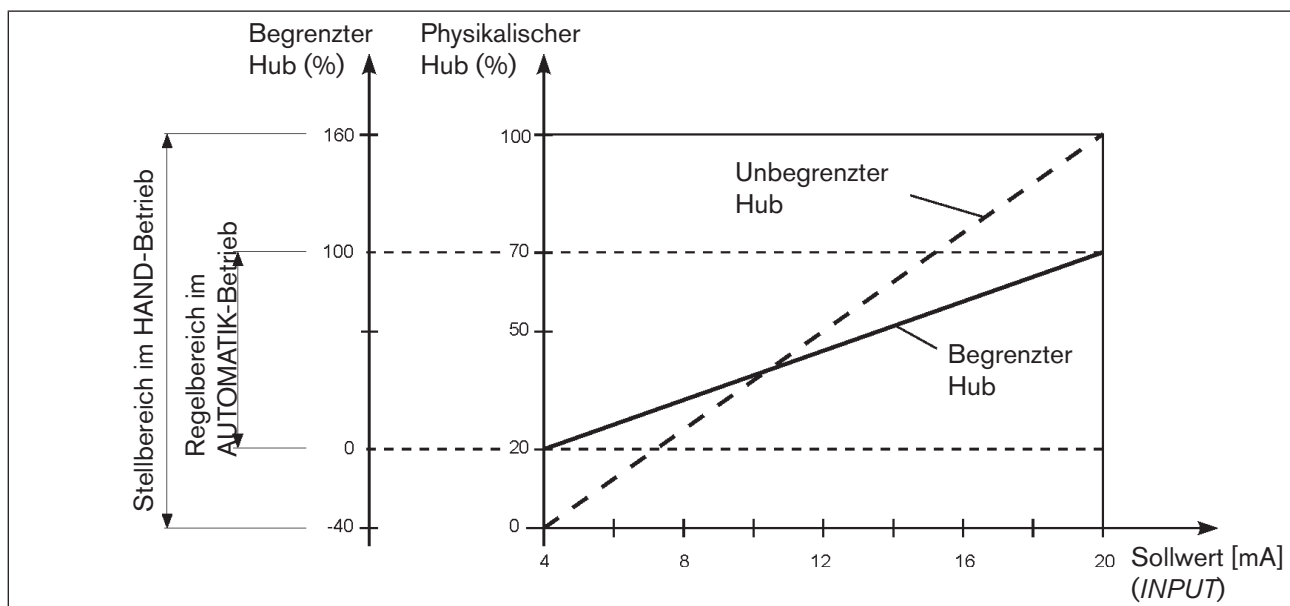
Bild 55: Diagramm X.LIMIT
