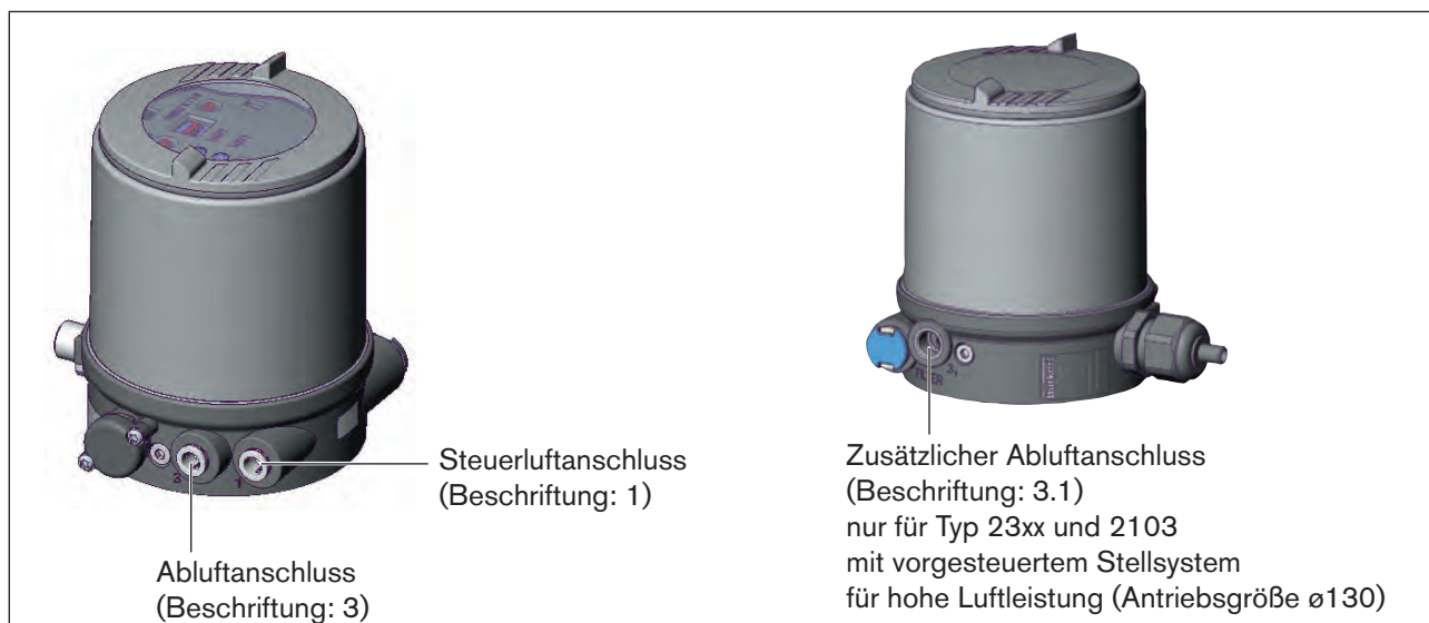
Bild 32: Pneumatischer Anschluss
