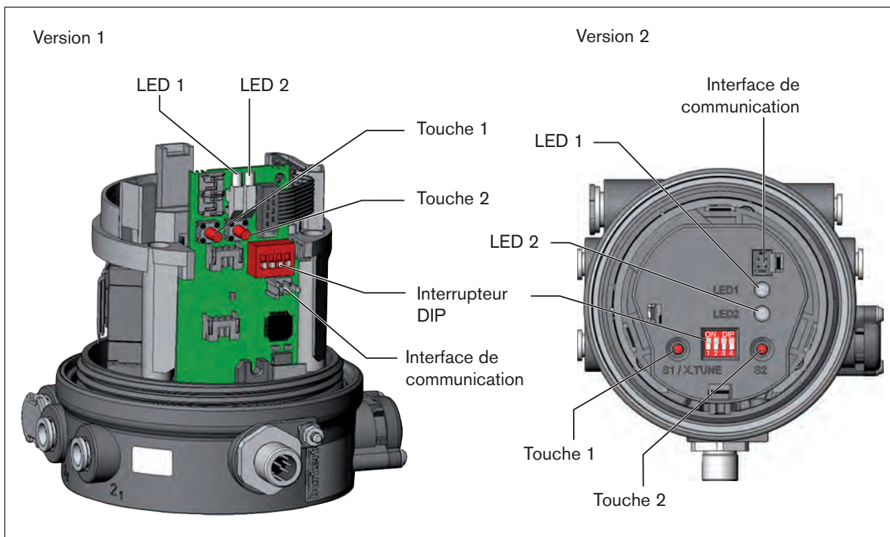
Figure 10 : Description des éléments de commande
